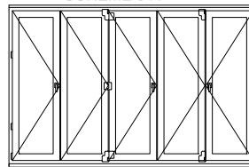
ESQUEMA 541/ SCHEME 541
