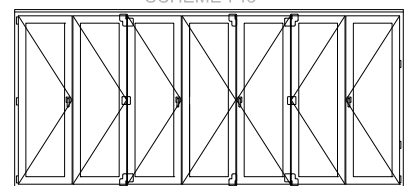
ESQUEMA 743/ SCHEME 743
