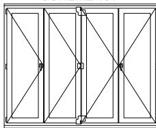
ESQUEMA 651/ SCHEME 651
