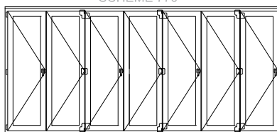
ESQUEMA 770/ SCHEME 770
