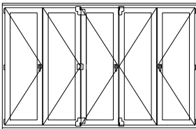
ESQUEMA 761/ SCHEME 761
